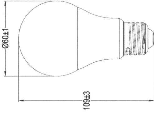
寸法図
